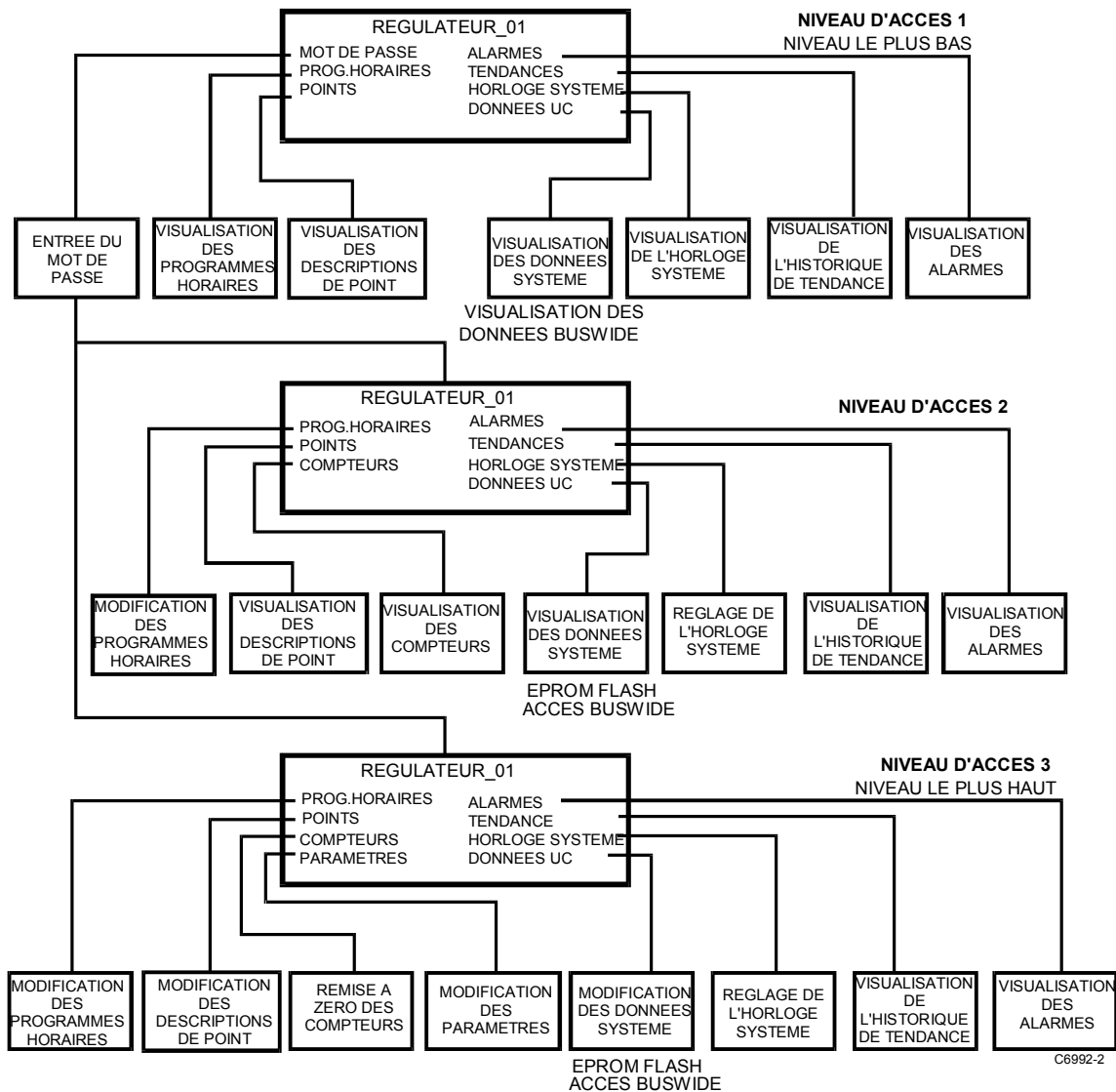
Résumé des fonctions du XI581/2 correspondant aux différents niveaux d'accès.
